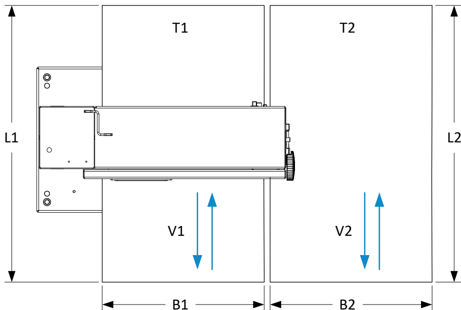
Figuur: Afkortzaag met tafels T1 en T2 (bovenaanzicht)
